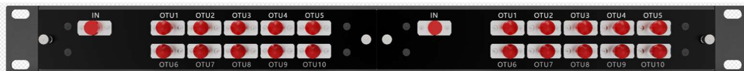
1U 2槽位机箱，可插2个分光器模块
