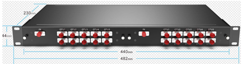
1U 2槽 机箱
